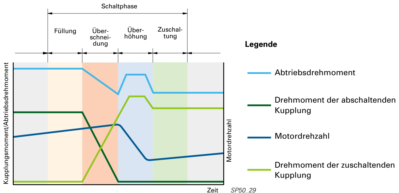
Momenten- und Motordrehzahlverlauf bei einer Zug-Hochschaltung
