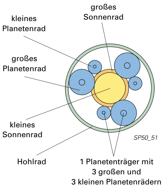
Ravigneaux-Planetenradsatz
