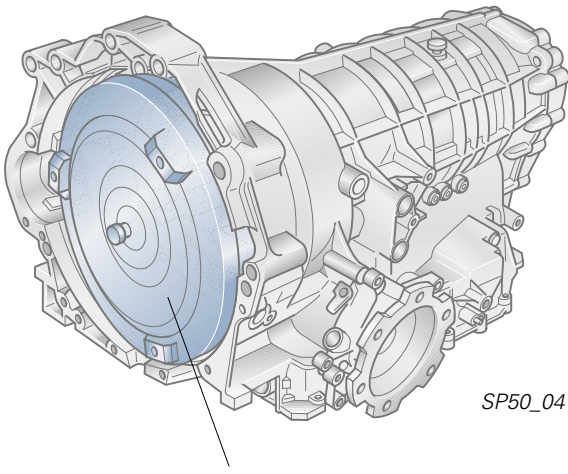
Drehmomentwandler
